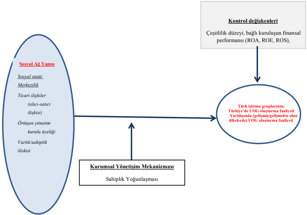
Şekil 1. Araştırma Tasarımı
